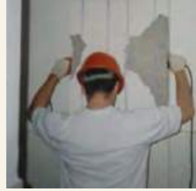
Görüntü 14. Yer ile yapının deprem öncesinde davranışını belirlemek için yapılan yer-yapı jeofiziği çalışmalarından birkaç örnek. Yukarıda çalkalanma(rezonans) ölçümü, ortada yer ıslaklığı için elektro çekimi, aşağıda beton niteliği için ultrason.
