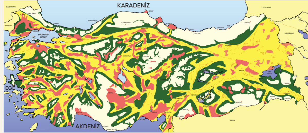
Görüntü 1. Türkiye'nin Deprem ile Etkileme Bölgeleri, (2005).
